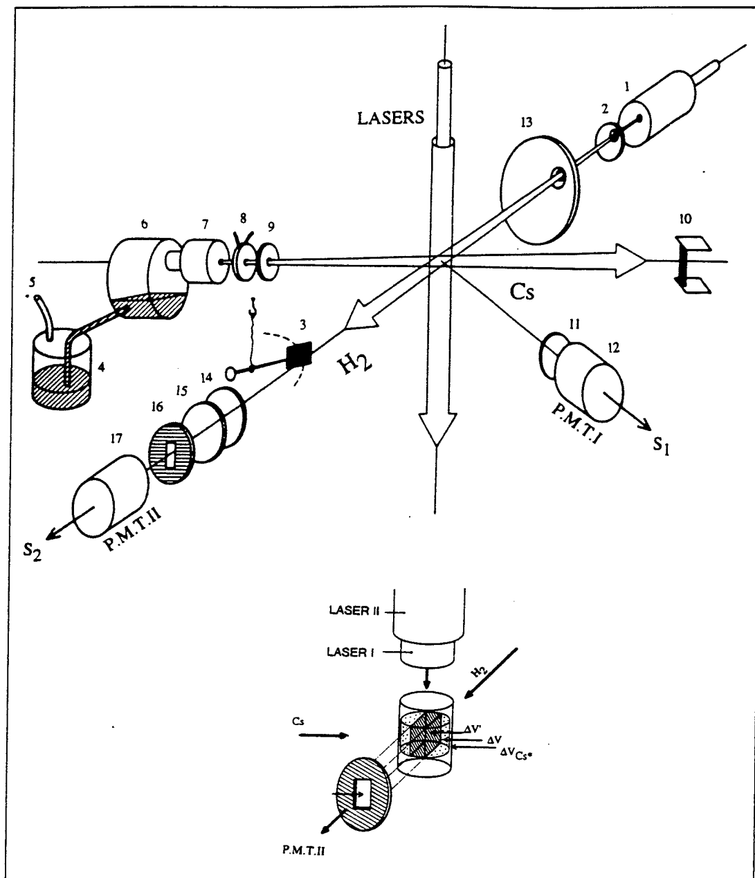
Figure 4.1: Schéma de l'expérience. Jet supersonique d'hydrogène : (1) tuyère, (2) écorceur, (3) pendule de torsion. Jet de césium : (4) réservoir, (5) pression d'argon, (6) première chambre, (7) deuxième chambre et tuyère, (8) diaphragme refroidi, (9) diaphragme, (10) fil chaud. Fluorescence des atomes de césium : (11) filtre, (12) photomultiplicateur P.M.I. Fluorescence des produits CsH : (13) miroir parabolique, (14) filtres réjecteurs infrarouge, (15) lentille, (16) diaphragme, (17) photomultiplicateur refroidi P.M.II. Dans la partie inférieure les volumes de collision: \Delta V_{\text{Cs}^*} est la zone de fluorescence du jet de césium, \Delta V est le volume de collision effectif et \Delta V' est le volume de détection vu par le P.M.II à travers le diaphragme (16).
