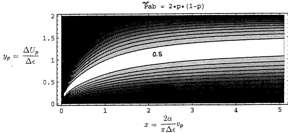
Figure 5.11: Probabilité de transition |a\rangle \rightarrow |b\rangle moyenne, \tilde{P}_{ab} = 2p(1-p) , pour deux passages dans la région d'interaction en R = R_p . L'axe x est proportionnel à la vitesse radiale v_p et y_p à l'écart des états adiabatiques en R_p (courbes de niveaux espacées de 0,05).
