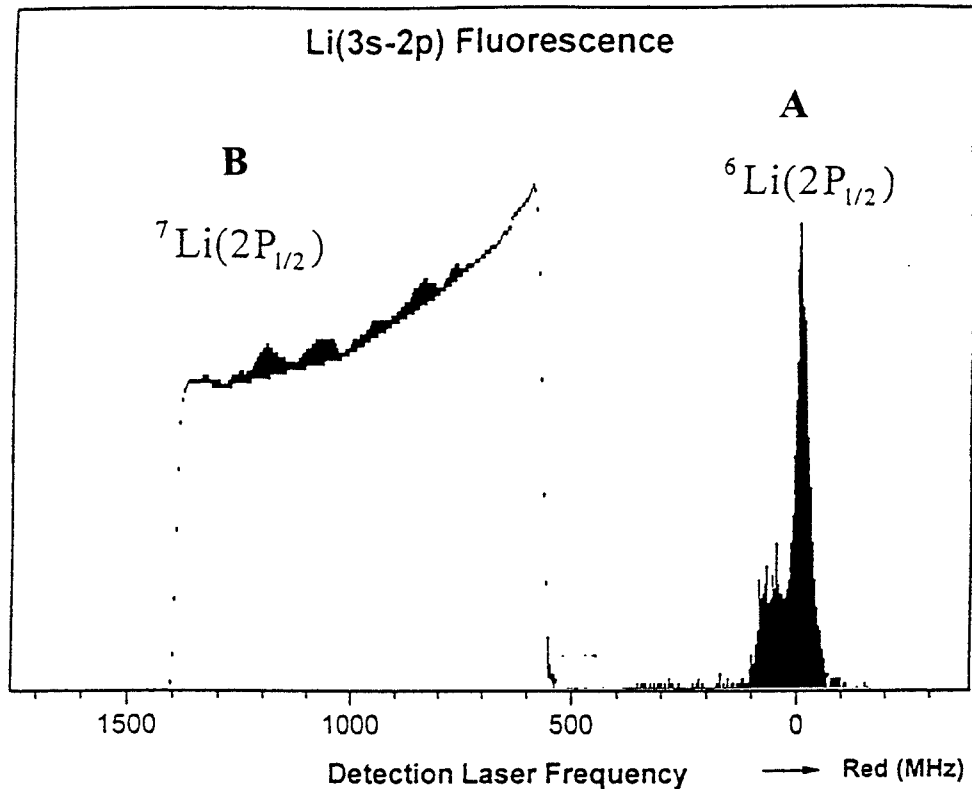
Figure 6.7: (Manip 694 B) Le laser excitateur I peuple le niveau {}^6\text{Li}(2P_{1/2}) . Spectre A: Le laser de détection II balaye la transition {}^6\text{Li}(2P_{1/2}) \rightarrow 3S_{1/2} . On obtient la fluorescence directe: F(\text{directe}) . Spectre B: Le laser de détection balaye la transition {}^7\text{Li}(2P_{1/2}) \rightarrow 3S_{1/2} . On obtient la fluorescence de transfert: F(\text{transfert}) .
