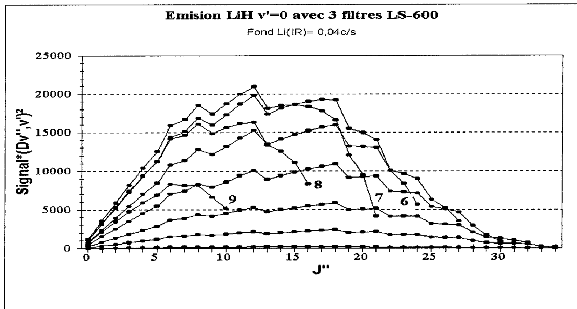
Figure 3.14: Evaluation du signal de fluorescence de LiH attendue avec 3 filtres LS-600 compte tenu de la probabilité de pompage |D(R)|^2 (en pompage faible).
