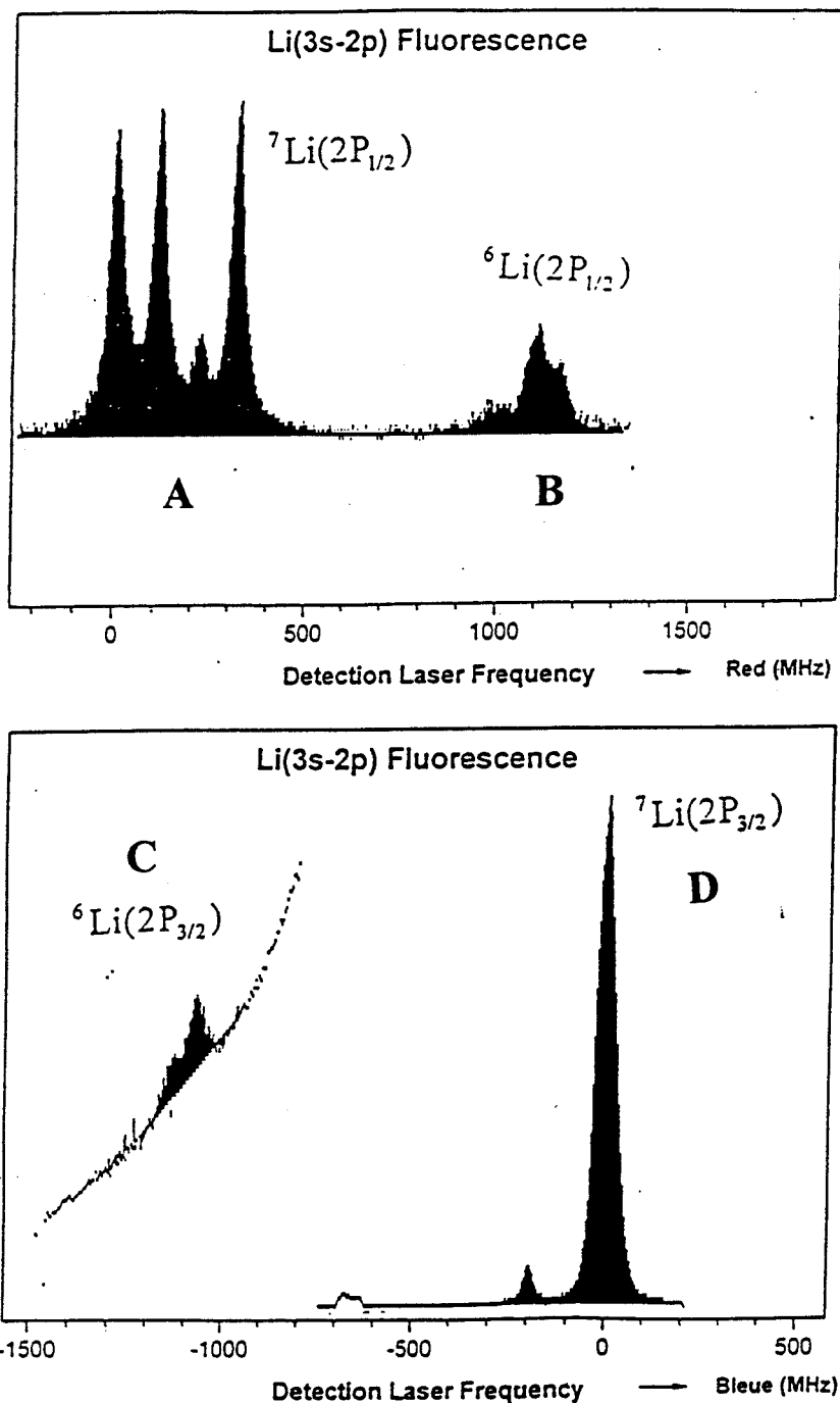
Figure 6.6: Le laser exciteur I peuple le niveau {}^7\text{Li}(2P(3/2)) . Spectre D : (Manip 701 et 702 B) Le laser de détection II balaye la transition {}^7\text{Li}(2P(3/2) \rightarrow 3S(1/2)) . On obtient la fluorescence directe: F_D (directe). Spectre C : Le laser de détection II balaye la transition {}^6\text{Li}(2P(3/2) \rightarrow 3S(1/2)) . On obtient la fluorescence de transfert: F_C (transfert). Spectre A : (Manip 699 A et 700) Le laser de détection II balaye la transition {}^7\text{Li}(2P(1/2) \rightarrow 3S(1/2)) . On obtient la fluorescence de transfert: F_A (transfert). Spectre B : Le laser de détection II balaye la transition {}^6\text{Li}(2P(1/2) \rightarrow 3S(1/2)) . On obtient la fluorescence de transfert: F_B (transfert).
