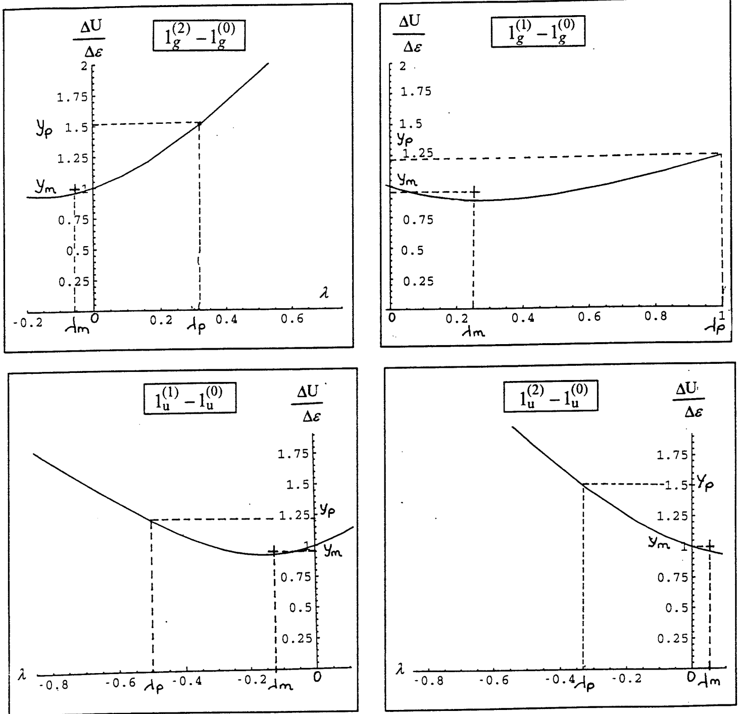
Figure 5.13: Couplage radial 1_\omega - 1_\omega . Les différences d'énergie \Delta U(1_\omega) sont représentées en fonction de \lambda = \omega R_o^3 / R^3 . On a indiqué dans chaque cas la valeur de \lambda_p qui correspond au milieu de la région d'interaction et la valeur de \lambda_m utilisée pour le calcul des paramètres de couplage.
