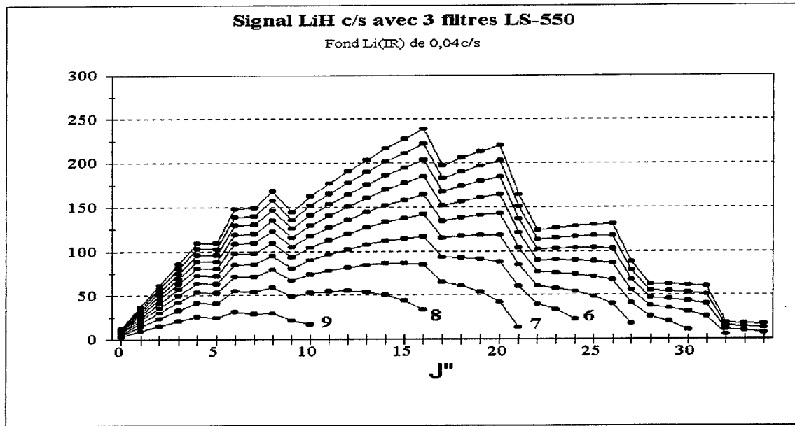
Figure 3.11: Evaluation du signal de fluorescence de LiH attendue avec 3 filtres LS-550 en saturation de pompage (en supposant que tous les produits LiH sont détectés avec la même efficacité).
