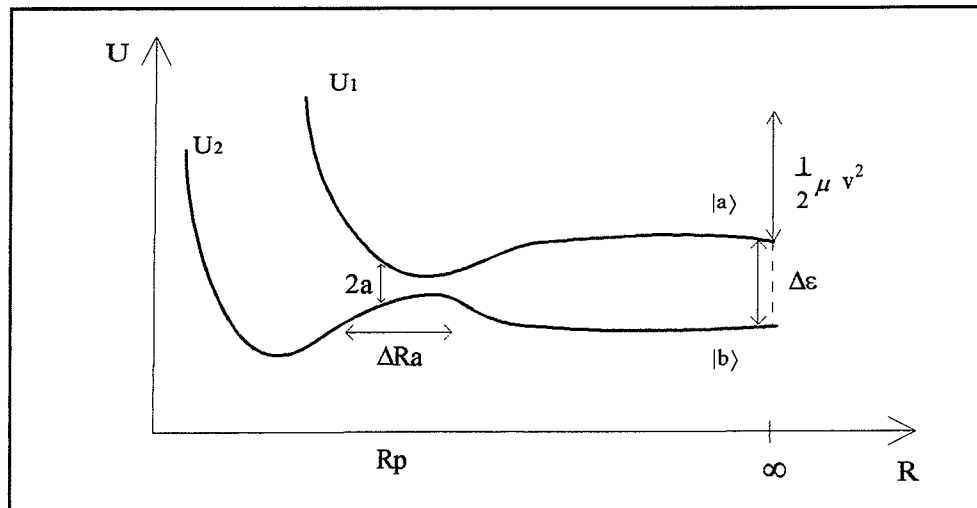
Figure 5.5: Energie des états adiabatiques. R_p est le centre de la zone de couplage.
