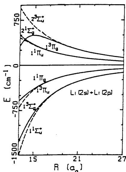
Figure 5.19: Energies potentielles des états de Li_2 issus à l'infini de Li(2s)+Li(2p) . Les états avec symétrie "ungerade" sont représentés en pointillé.
