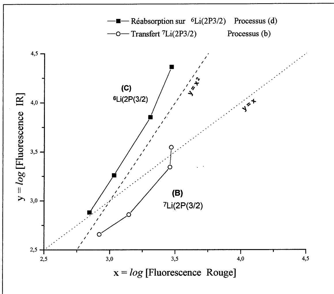
Figure 6.12: (Manip 585) Evolution du nombre de transfert {}^7\text{Li}(2P(3/2) \rightarrow 2P(1/2)) (processus (b)) et de réabsorption par {}^6\text{Li} (processus (d)) avec la densité n_o du jet de lithium. La puissance du laser I d'excitation reste constante et la puissance absorbée est faible (5-10%). Si on suppose que la fluorescence rouge, F_R , varie proportionnellement à la densité n_o du jet, les processus (b) et (d) (fluorescences des pics B et C) doivent varier comme F_R^2 \propto n_o^2 . Ceci est bien vérifié pour le processus (d) de réabsorption par {}^6\text{Li} et assez bien pour le processus (b).
