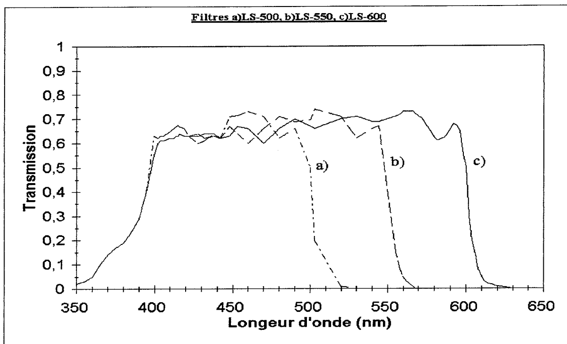
Figure 3.6: Courbes de transmission des filtres utilisés: (a)LS-500,(b)LS-550,(c)LS-600
