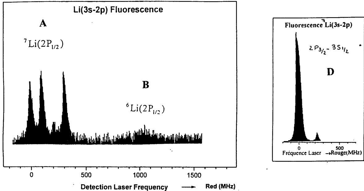
Figure 6.4: (Manip 670 A) Le laser excitateur I peuple le niveau {}^7\text{Li}(2P(3/2)) . Spectre D : Le laser de détection II balaye les transitions {}^7\text{Li}(2P(3/2) \rightarrow 3S(1/2)) . On obtient la fluorescence directe: F(\text{directe}) . Spectre A : Le laser de détection balaye la transition {}^7\text{Li}(2P(1/2) \rightarrow 3S(1/2)) . On obtient la fluorescence de transfert: F(\text{transfert}) . Spectre B : Le laser de détection balaye la transition {}^6\text{Li}(2P(1/2) \rightarrow 3S(1/2)) .
