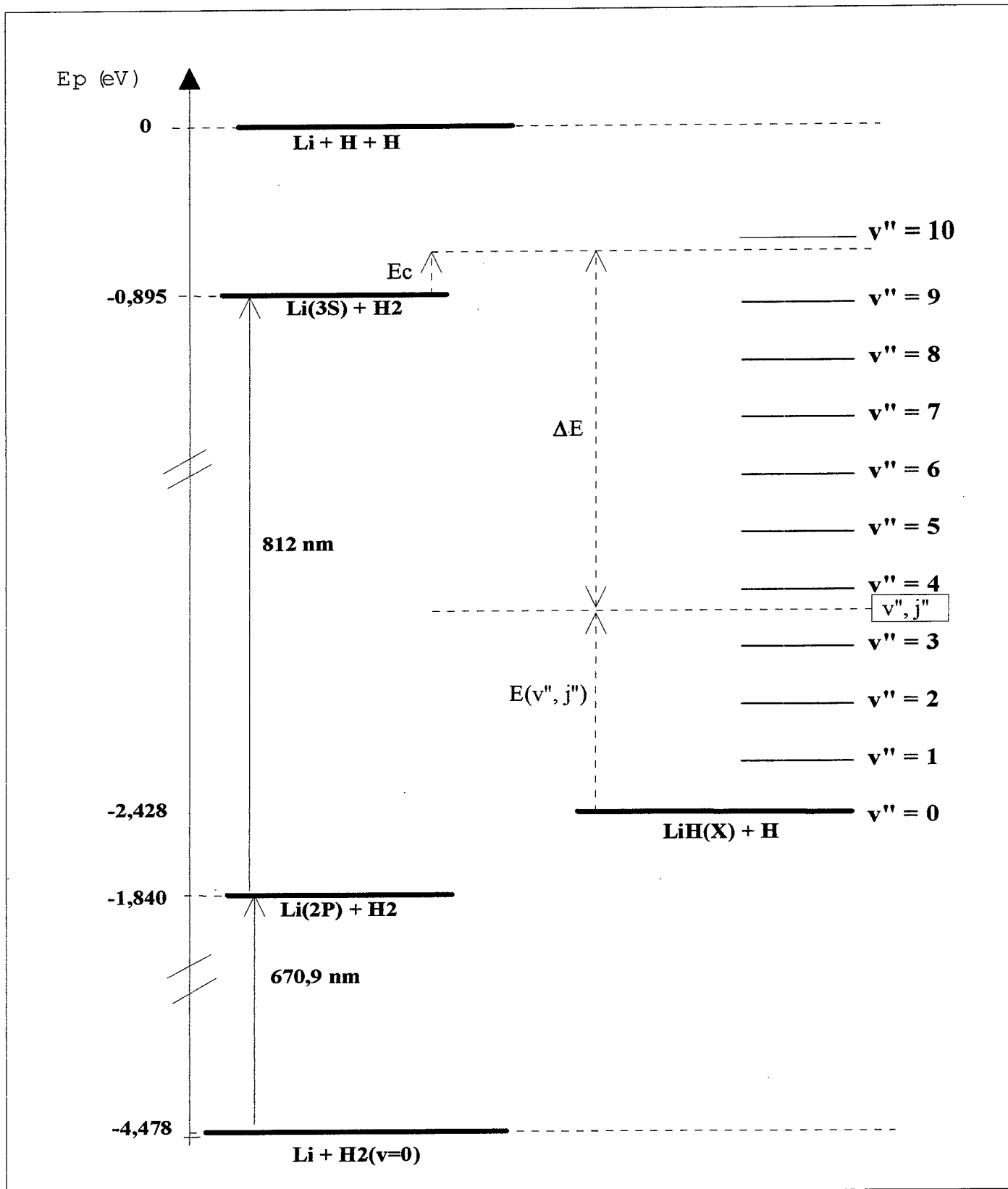
Figure 2.4: Bilan énergétique de la réaction \text{Li}(3S) + \text{H}_2 \rightarrow \text{LiH} + \text{H}
