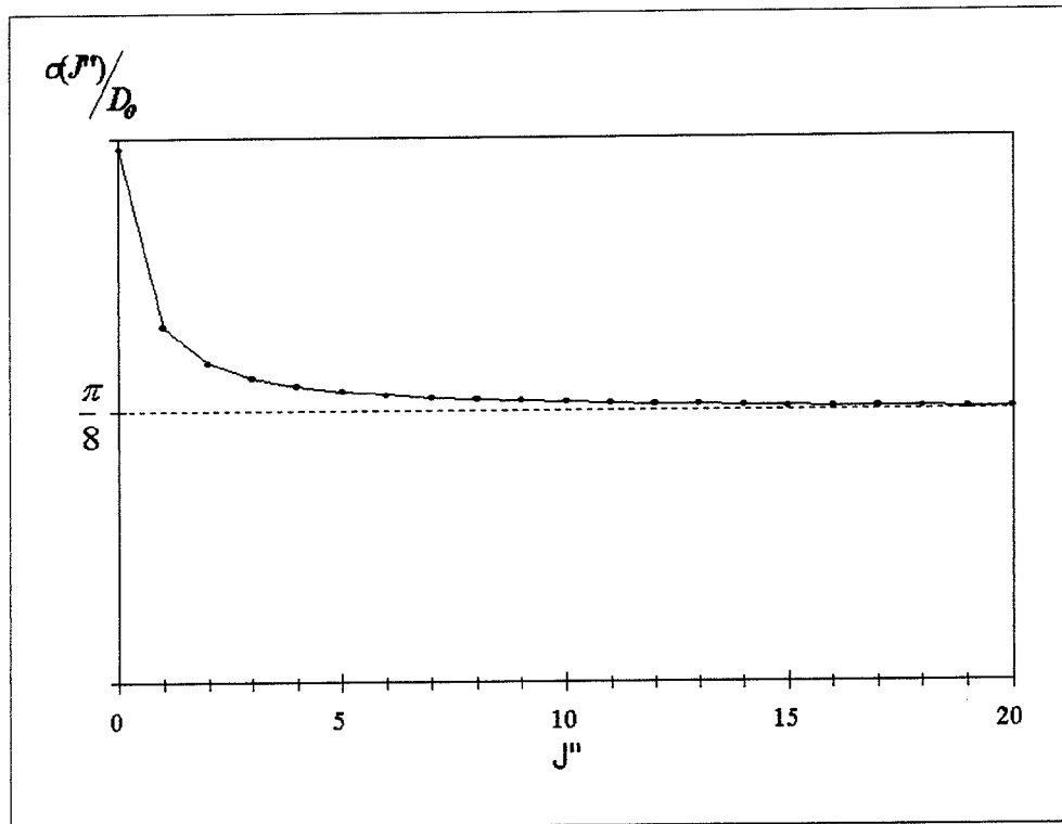
Figure 3.19: Calcul de \sigma(J'')/D_0 pour la transition de LiH X^1\Sigma^+(v''=7, J'') \rightarrow A^1\Sigma^+(v'=0, J'=J''+1) .
