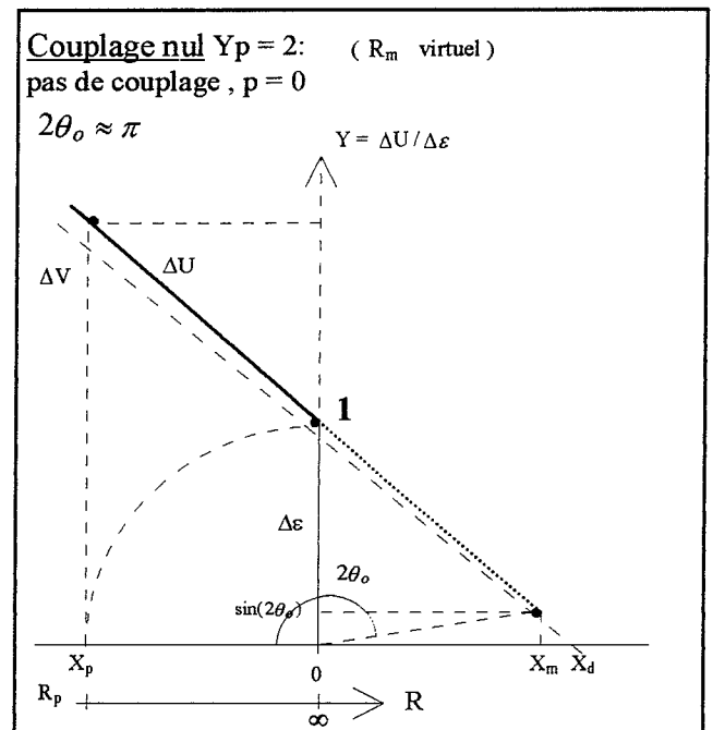
Figure 5.8: Modèle exponentiel. On a représenté Y = \Delta U/\Delta\epsilon en fonction de l'interaction X = \exp(-\alpha(R-R_p)) . La force du couplage est liée au rapport Y_p = \Delta U_p/\Delta\epsilon , où \Delta U_p est l'écart des termes adiabatiques au centre de la région d'interaction en R = R_p . Quatre cas de couplage exponentiel. Couplage fort (passage diabatique), couplage moyen (cas quasiparallèle), couplage faible (passage adiabatique) et couplage nul.
