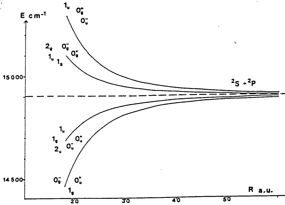
Figure 5.20: Energies potentielles des 16 états \Omega_{u,g} de Li_2 issus de Li(2s)+Li(2p)
