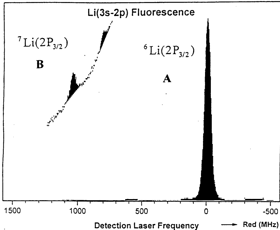
Figure 6.9: (Manip 703B) Le laser exciteur I sur {}^6\text{Li}[(2S(1/2), F'=3/2) \rightarrow (2P(3/2))] . Spectre A : Le laser de détection II balaye la transition {}^6\text{Li}(2P(3/2) \rightarrow 3S(1/2)) . On obtient la fluorescence directe: F(\text{directe}) . Spectre B : Le laser de détection II balaye la transition {}^7\text{Li}(2P(3/2) \rightarrow 3S(1/2)) . On obtient la fluorescence de transfert: F(\text{transfert}) .
