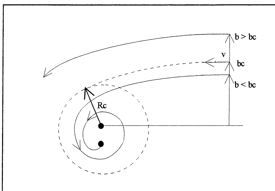
Figure 5.15: Schéma du paramètre d'impact de capture b_c .
