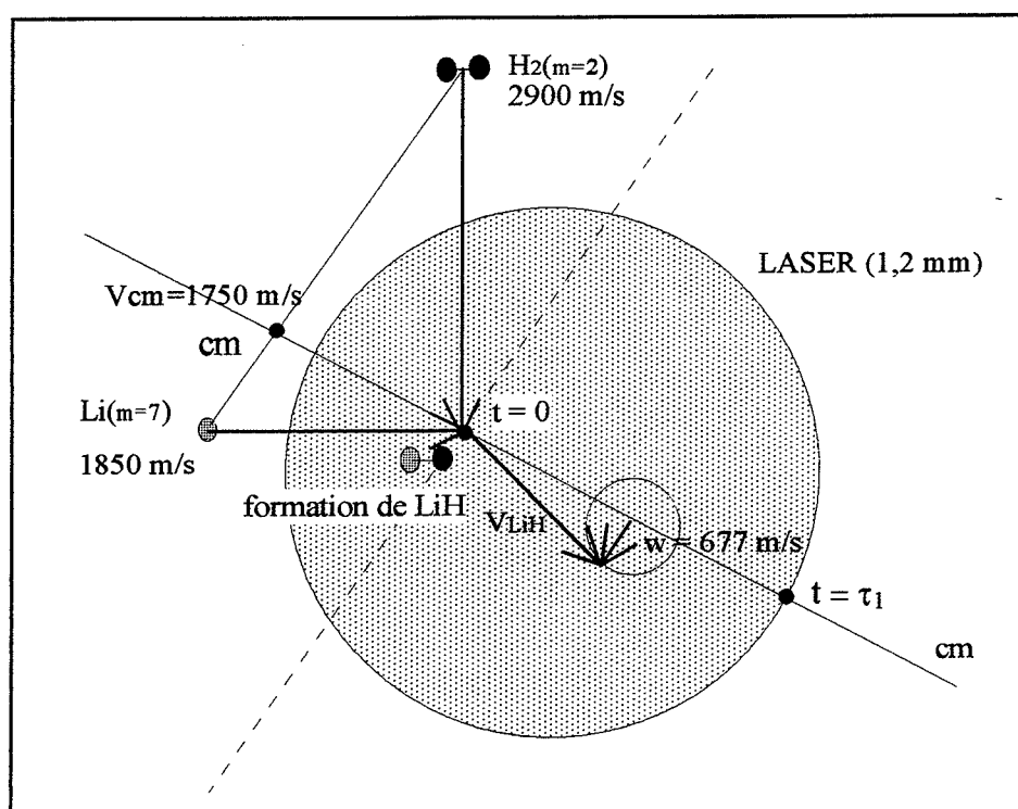
Figure 3.18: Représentation schématique de l'interaction laser-molécule. LiH est formé au temps t=0 . Le temps \tau_1 est le temps d'interaction de la molécule LiH avec le faisceau laser.
