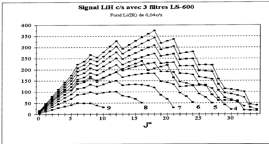
Figure 3.13: Evaluation du signal de fluorescence de LiH attendue avec 3 filtres LS-600 en saturation de pompage (en supposant que tous les produits LiH sont détectés avec la même efficacité).
