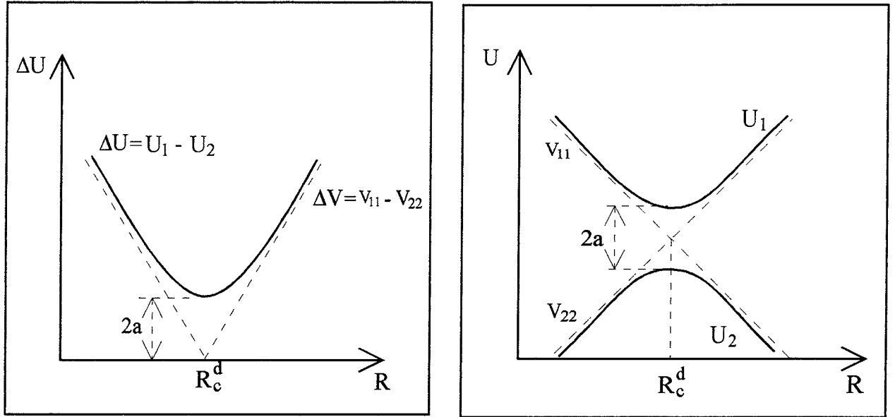
Figure D.1: Modèle linéaire. Energies adiabatiques U_1 et U_2
