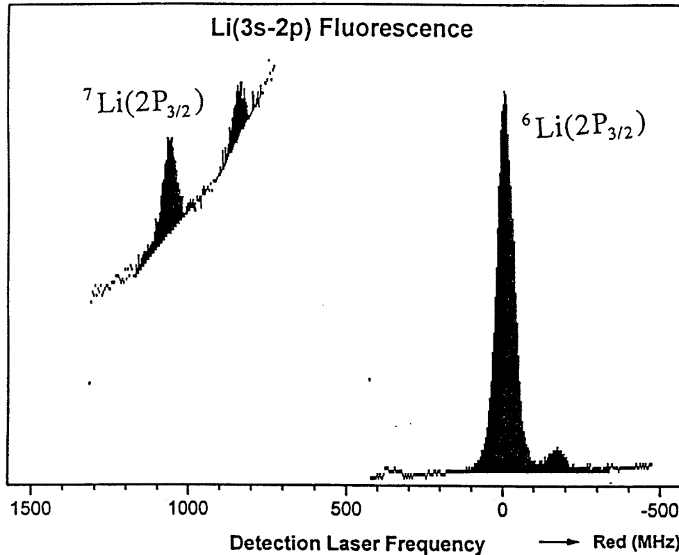
Figure 6.10: (Manip 705B) Le laser excitateur I sur {}^6\text{Li}[2S_{1/2}, F'' = 1/2 \rightarrow 2P_{3/2}, F' = 1/2, 3/2] qui est coïncidente (à 29 MHz près) avec la transition {}^7\text{Li}[2S_{1/2}, F'' = 2 \rightarrow 2P_{1/2}, F' = 1] . Spectre A : Le laser de détection II balaye la transition {}^6\text{Li}(2P(3/2) \rightarrow 3S(1/2)) . On obtient la fluorescence directe: F(\text{directe}) . Spectre B : Le laser de détection II balaye la transition {}^7\text{Li}(2P(3/2) \rightarrow 3S(1/2)) . On obtient la fluorescence de transfert: F(\text{transfert}) .
