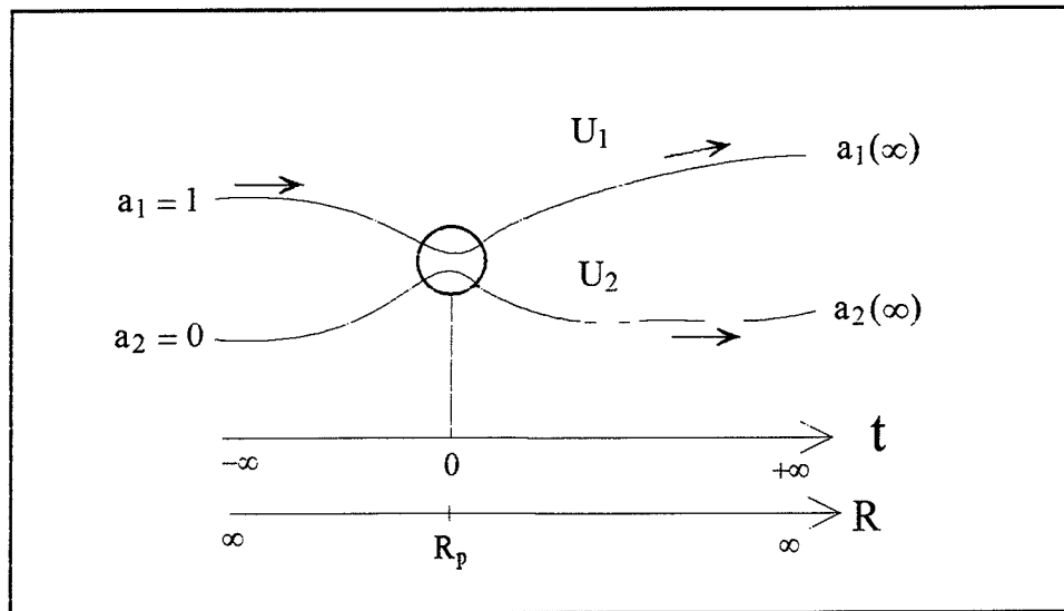
Figure 5.10: Modèle exponentiel. Evolution des amplitudes sur les états adiabatiques dans la région de couplage, t = 0 est l'instant de passage dans la région de pseudo-croisement R = R_p
