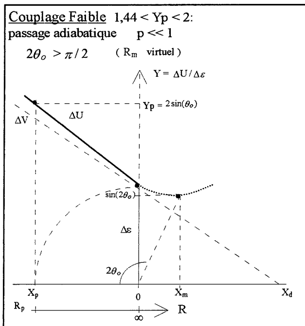
Figure 5.8: Modèle exponentiel. On a représenté Y = \Delta U/\Delta\epsilon en fonction de l'interaction X = \exp(-\alpha(R-R_p)) . La force du couplage est liée au rapport Y_p = \Delta U_p/\Delta\epsilon , où \Delta U_p est l'écart des termes adiabatiques au centre de la région d'interaction en R = R_p . Quatre cas de couplage exponentiel. Couplage fort (passage diabatique), couplage moyen (cas quasiparallèle), couplage faible (passage adiabatique) et couplage nul.
