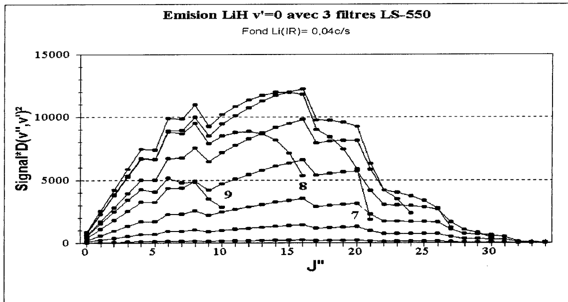
Figure 3.12: Evaluation du signal de fluorescence de LiH attendue avec 3 filtres LS-550 compte tenu de la probabilité de pompage |D(R)|^2 (en pompage faible).
