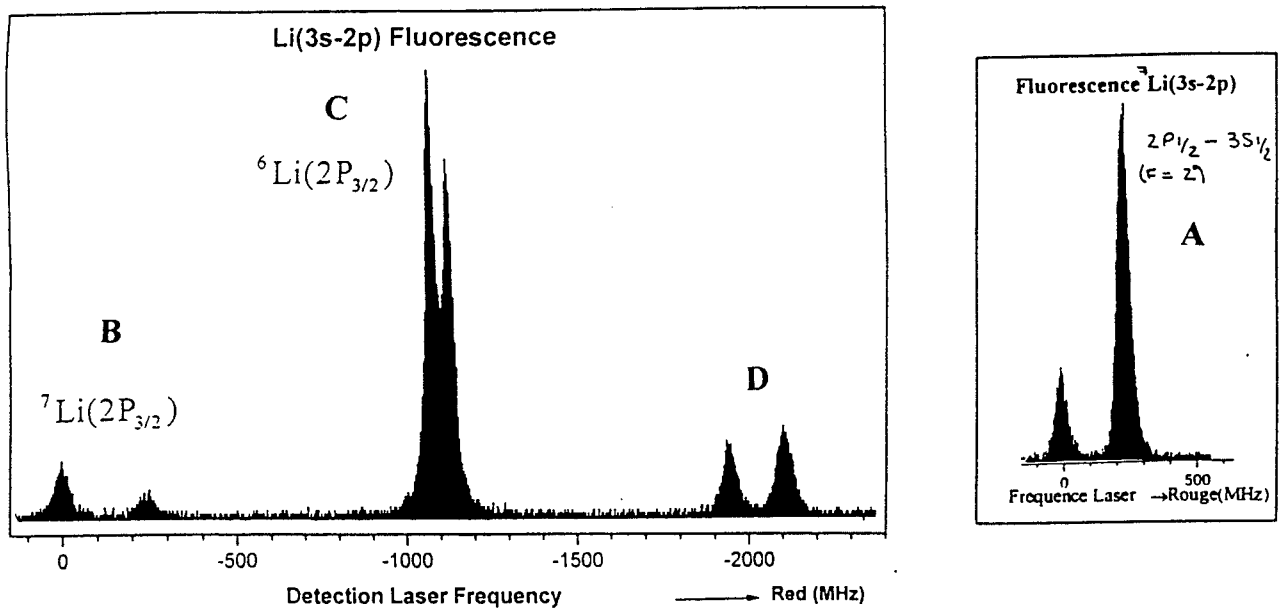
Figure 6.5: (Manip 672 A, 671) Le laser exciteur I peuple le niveau {}^7\text{Li}(2P(1/2)) . Spectre A : Le laser de détection II balaye la transition {}^7\text{Li}(2P(1/2) \rightarrow 3S(1/2)) . On obtient la fluorescence directe: F(\text{directe}) . Spectre B : Le laser de détection II balaye la transition {}^7\text{Li}(2P(3/2) \rightarrow 3S(1/2)) . On obtient la fluorescence de transfert: F(\text{transfert}) . Spectre C : Le laser de détection II balaye la transition {}^6\text{Li}(2P(3/2) \rightarrow 3S(1/2)) . On obtient la fluorescence de transfert: F(\text{transfert}) . Spectre D : Fluorescence d'atomes {}^6\text{Li}(3S(1/2)) produits par un mécanisme à deux photons très proches de la résonance.
