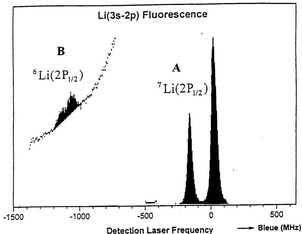
Figure 6.8: (Manip 706 A) Le laser exciteur I peuple le niveau {}^7\text{Li}(2P(1/2)) (composante 2). Spectre A : Le laser de détection II balaye la transition {}^7\text{Li}(2P(1/2) \rightarrow 3S(1/2)) . On obtient la fluorescence directe: F(\text{directe}) . Spectre B : Le laser de détection II balaye la transition {}^6\text{Li}(2P(1/2) \rightarrow 3S(1/2)) . On obtient la fluorescence de transfert: F(\text{transfert}) .
