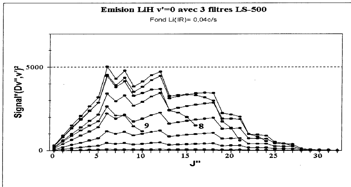
Figure 3.10: Evaluation du signal de fluorescence de LiH attendue avec 3 filtres LS-500 compte tenu de la probabilité de pompage |D(R)|^2 (en pompage faible).
