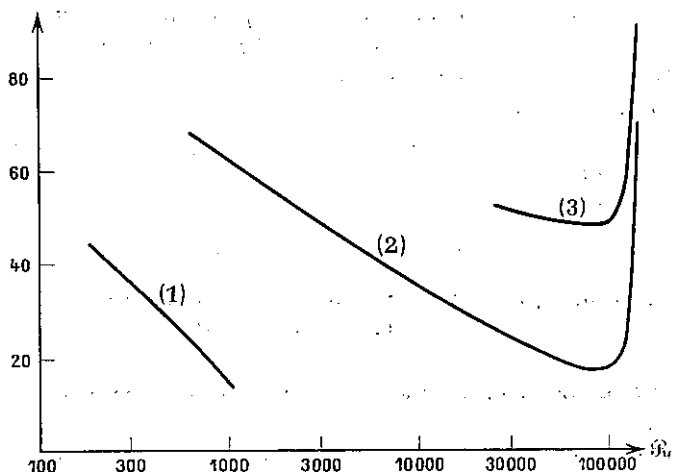
FIG. 58. — En abscisse, résolution \mathcal{R} ; en ordonnée, gain de luminosité. Courbe (1) : le réseau ( 65 \times 76 mm, \varphi = 30^\circ , \beta = 1/50 ) + un F. P. ; courbe (2) : le réseau + deux F. P. ; courbe (3) : le réseau + trois F. P.
