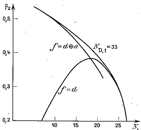
FIG. 37. — Variation du facteur \rho_2 en fonction de la finesse d'appareil; la courbe supérieure correspond aux meilleures conditions d'utilisation.
