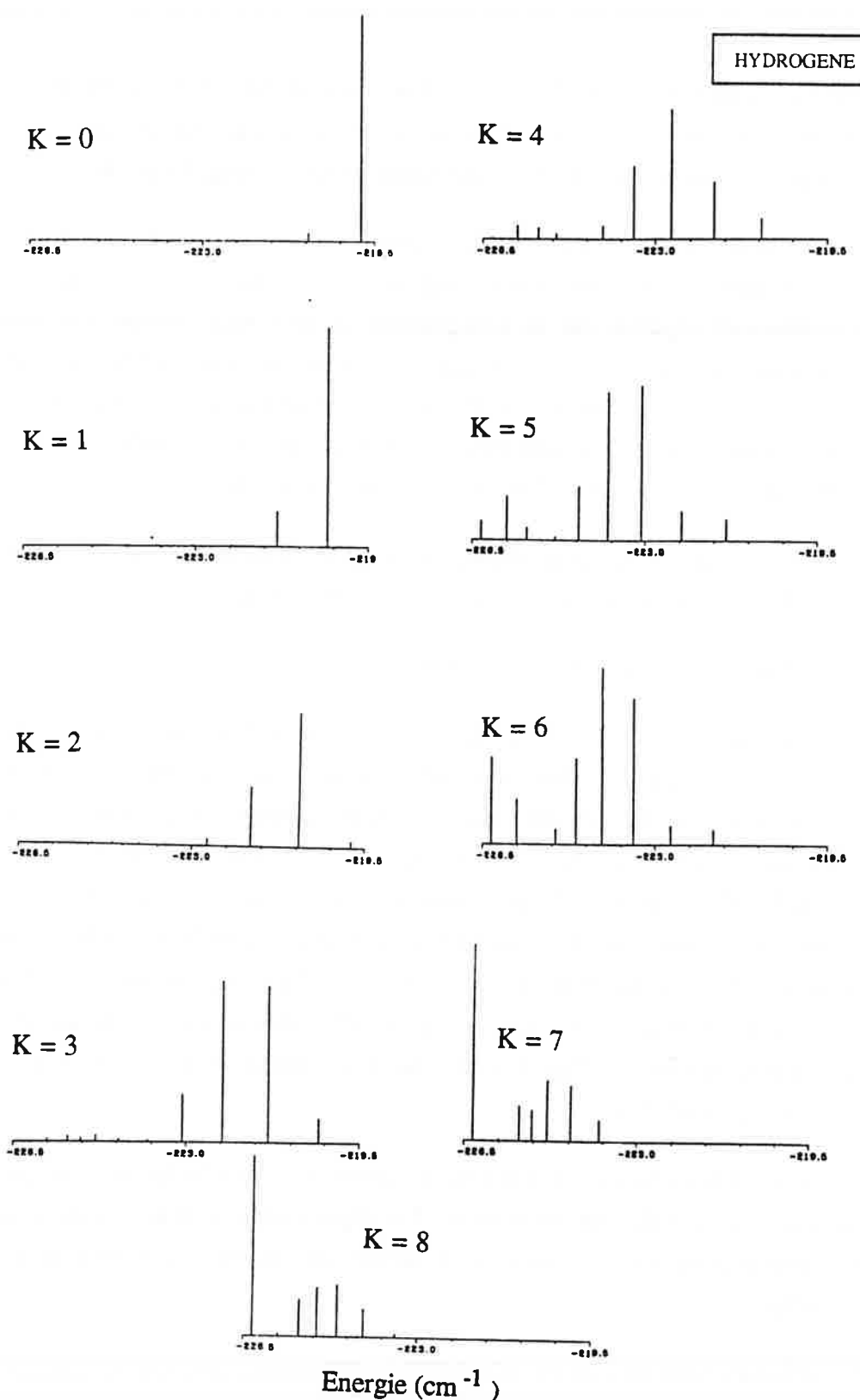
FIG (II.6) Répartition de la force d'oscillateur sur les états diamagnétiques du multiplet ( n = 22 M = 0 ) de l'hydrogène ( B = 5T ) en fonction de la symétrie de l'état relais ( n = 10 M = 1 K )
